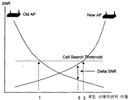
(그림 8) 단말의 로밍 시점
