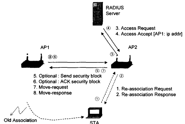
(그림 9) IAPP 동작 과정
