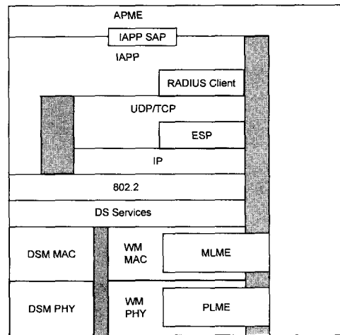
(그림 7) IAPP 구조도
