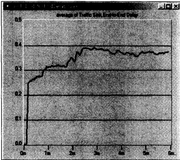
(그림 19) End-to-End Delay 측정(기준)
