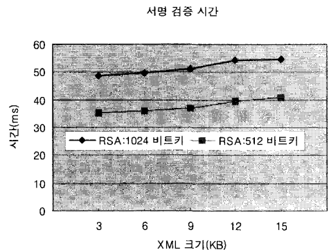
(b) M의 크기에 따른 서명 검증시간
