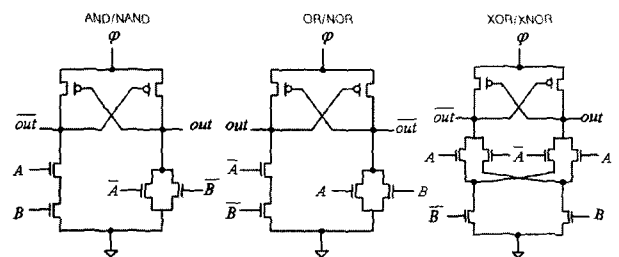
그림 3. AND 게이트, OR 게이트와 exclusive-OR 게이트 Fig. 3. ECRL AND gate, OR gate and exclusive-OR gate.
