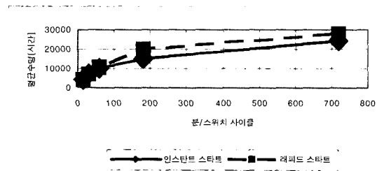
그림 7. 사용주기에 따른 형광램프의 평균수명 변화
