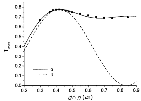
그림 6. 유전율 이방성이 양인 액정을 사용한 FFS 모드의 위상지연값 변화에 따른 투과율 최대값의 계산 결과.
