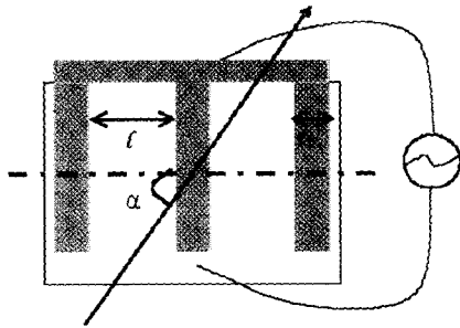
그림 2. FFS 모드의 정면에서 관찰한 셀 구조 개략도.
