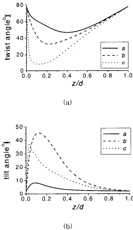
그림 5. 전극 위치별 액정 분자의 (a) twist 및 (b) tilt 각 분포.
