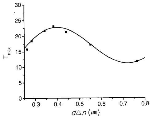
그림 7. 셀갭이 3.8 \mu\text{m} 인 경우 위상지연 변화에 따른 T_{\max} 측정값. 여기서, 실선은 식 (3)으로 fitting 결과이다.
