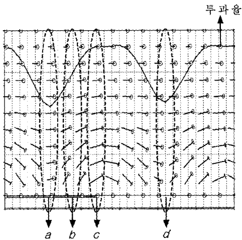
그림 3. 유전율 이방성이 양인 액정을 사용한 FFS 모드의 구동전압 인가상태에서의 액정 방향자의 분포.
