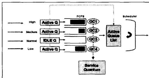
[그림 3] AIWFQ 구조(proposal algorithm) 새롭게 제안한 AIWFQ는 WFQ를 기반으로 하는
