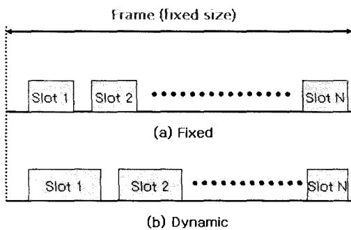
[그림 2] TDMA 기반의 고정(a)과 동적(b)대역할당 구조
