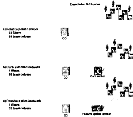
[그림 1] FTTH 구현을 위한 가입자 망 구성 시나리오
