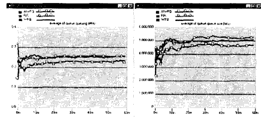
[그림 4.a] High Class 버퍼지연(L), 버퍼크기(R)
