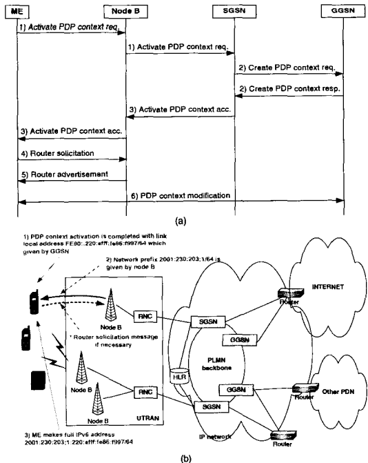
그림 5. 제안한 IPv6 stateless address autoconfiguration 과정
