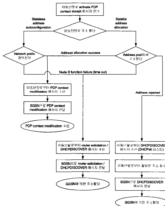
그림 10. 문제 발생시 Node B의 동작 플로우 차트
