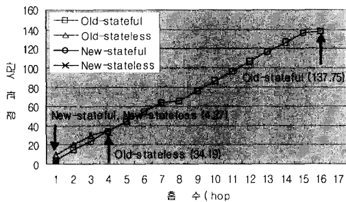
그림 12. 이동단말로의 IPv6 주소할당 시간
