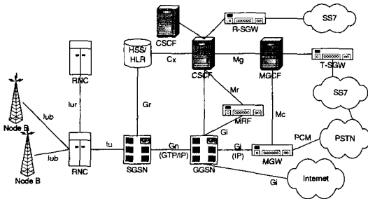
그림 1. 3GPP에서 정의한 IP 기반 이동통신망
