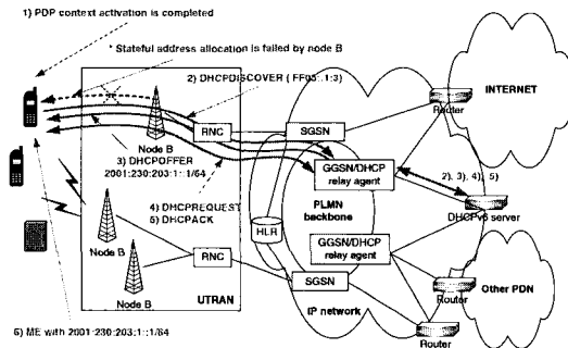
그림 9. IPv6 stateful address allocation 방식에서 라우팅 수정과정
