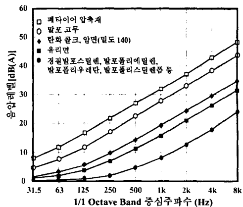
그림 3. 재료별 투과손실 산정결과 ("공동주택 바닥충격음 저감기술개발"(LG건설,1998)참조)
