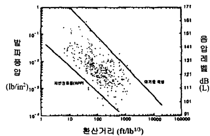
그림 1. 환산거리에 따른 발파소음 측정
