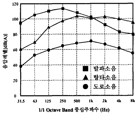
그림 2. 소음원에 따른 주파수특성 비교
