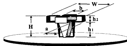
(a) 폴디드 멀티스트립 모노폴 안테나 (a) Folded multistrip monopole antenna
