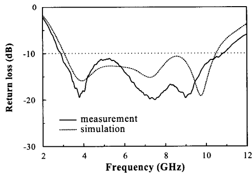
그림 6. 제작한 안테나의 반사손실 Fig. 6. Measured return loss.
