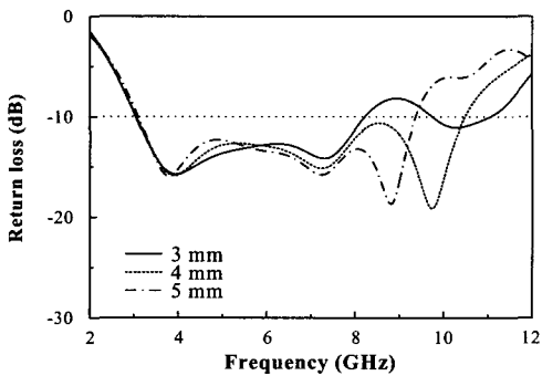
(b) a 에 따른 반사손실의 변화 (b) Return loss for different a
