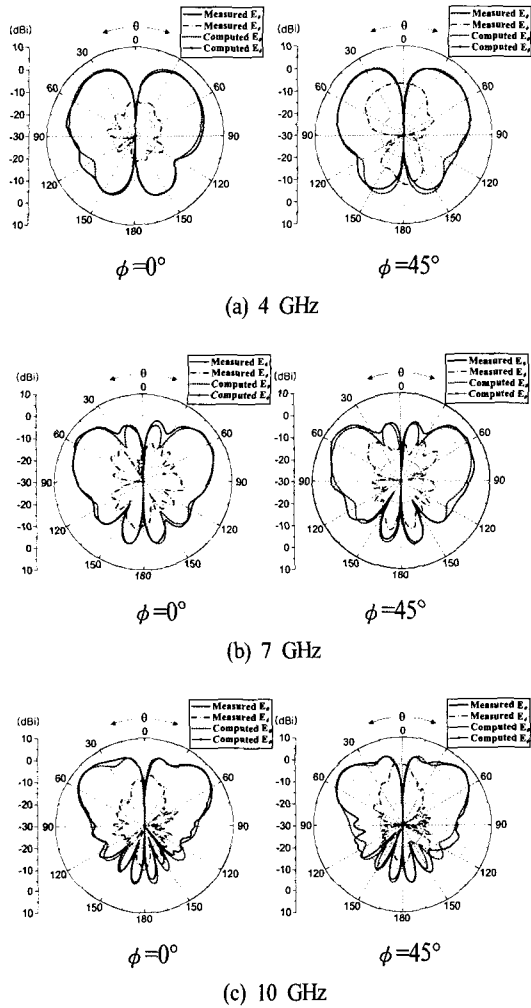
그림 7. 안테나 복사패턴 Fig. 7. Radiation pattern of antenna.
