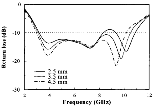
(c) h_2 에 따른 반사손실의 변화 (c) Return loss for different h_2
