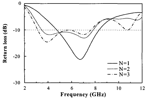
그림 2. N 에 따른 반사손실의 변화 Fig. 2. Return loss with respect to N .
