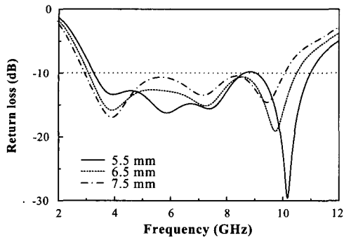
(a) h_1 에 따른 반사손실의 변화 (a) Return loss for different h_1
