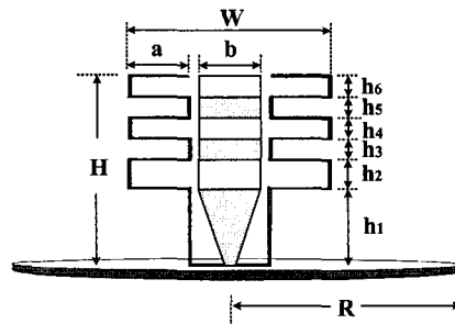
그림 3. 안테나의 설계변수 Fig. 3. Antenna design parameters.
