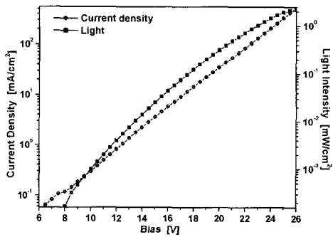
그림 8. 제작된 소자의 전류밀도-전압-광출력 특성. Fig. 8. Current density-voltage-light characteristics of the fabricated device.
