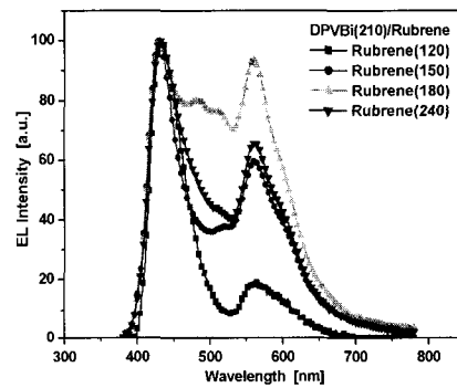
그림 6. Rubrene층의 두께 변화에 따른 EL 스펙트럼.
