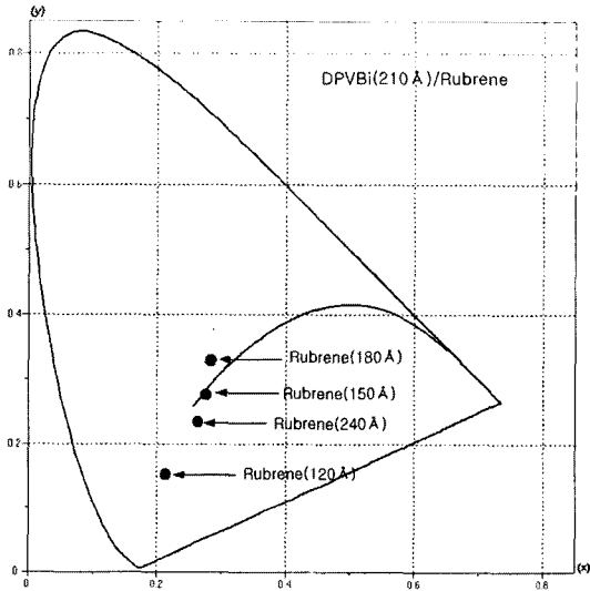
그림 7. Rubrene 층의 두께 변화에 따른 CIE 색좌표. Fig. 7. CIE coordinates of devices by varying the thickness of Rubrene layer.
