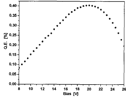
그림 9. 전압-외부양자효율 특성. Fig. 9. Voltage-external quantum efficiency characteristics.
