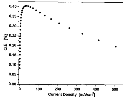
그림 10. 전류밀도-외부양자효율 특성. Fig. 10. Current density-external quantum efficiency characteristics.
