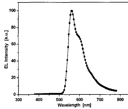
그림 3. ITO/NPB/Rubrene(150 Å)/BCP/Alq 3 /Al 구조의 소자에 대한 EL 스펙트럼. Fig. 3. EL spectrum of device having structure of ITO/NPB/Rubrene(150 Å)/BCP/Alq 3 /Al.
