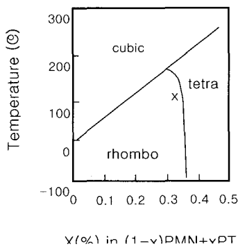
그림 2. PMN-PT 결정의 대칭구조. Fig. 2. Symmetry of PMN-PT crystals.
