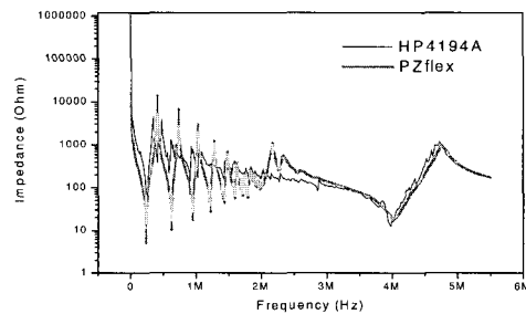
그림 9. RAD시편의 임피던스곡선. Fig. 9. Impedance spectrum of the RAD sample.
