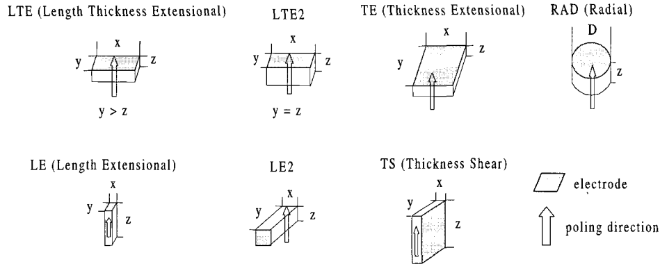
그림 3. 물성상수를 측정하기 위한 PMN-32%PT 시편형상.
