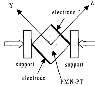
그림 4. LTE2시편을 이용한 c_{14}^E 측정.
