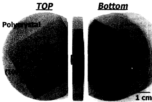
그림 1. 고상단결정법에 의한 PMN-PT 성장과정. Fig. 1. Process of PMN-PT growth by SSCG method.
