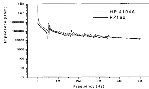
그림 7. LE2시편의 임피던스곡선 비교. Fig. 7. Impedance spectrum of the LE2 sample.
