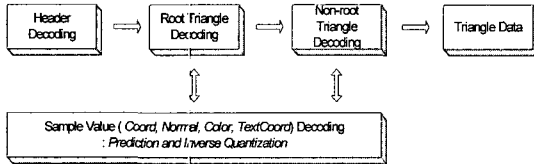
그림 6. Triangle data decoder의 블록도
