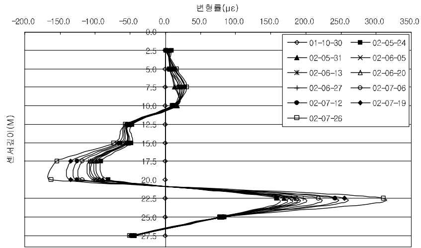
그림 7 3단 변형율 그래프.
