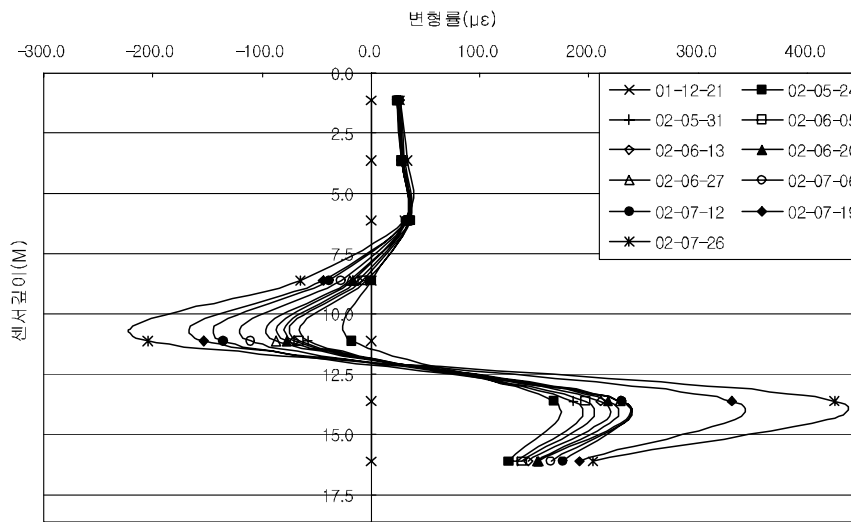
그림 5 1단 변형률 그래프.
