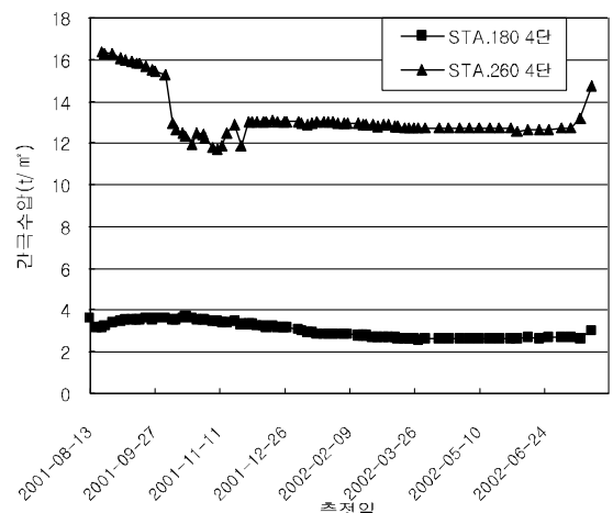
그림 10 4단 간극수압.
