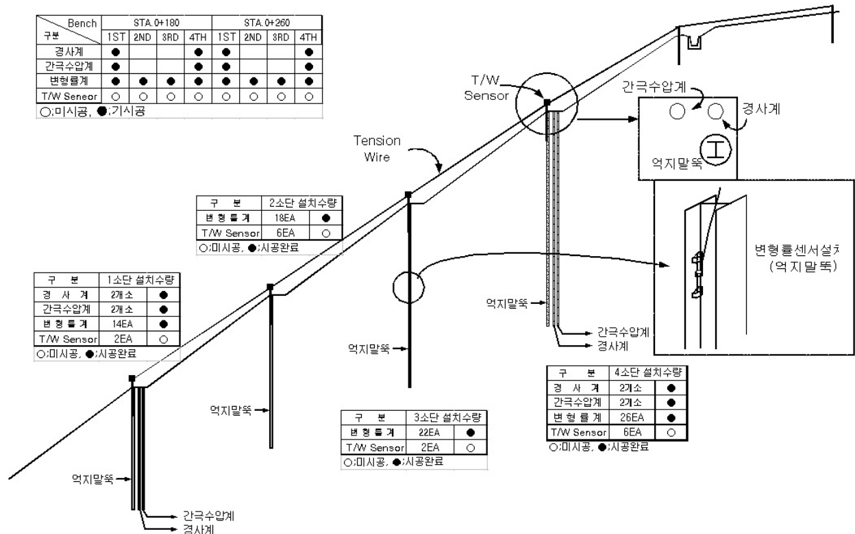
그림 1 계측기 설치 위치도.
