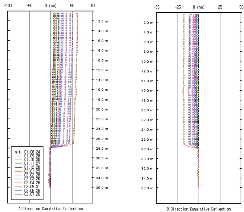
그림 4 4소단 월별 경사계 변위 추이.
