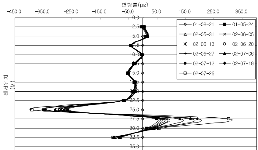
그림 8 4단 변형율 그래프.
