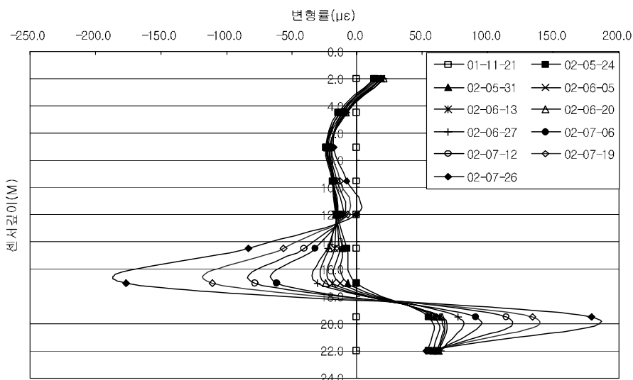
그림 6 2단 변형율 그래프.
