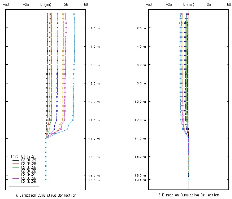
그림 3 1소단 월별 경사계 변위 추이.
