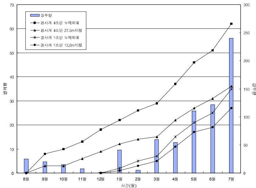
그림 2 월별 강우량 및 경사계 변위.
