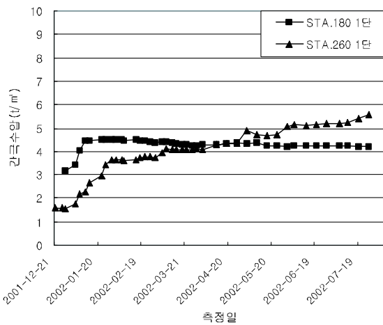
그림 9 1단 간극수압.
