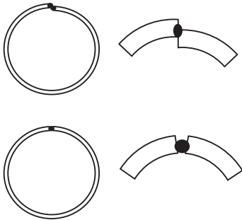
그림 3. Welding joints
