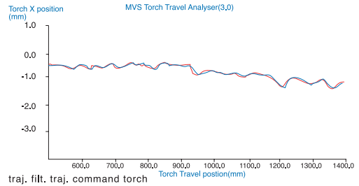
그림 14. Seam tracked welding line
