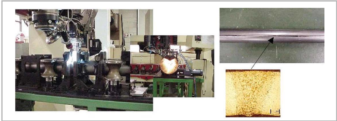
그림 17. Laser welded tube with good welding quality
