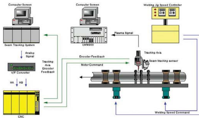
그림 11. Schematic diagram for construction and control
