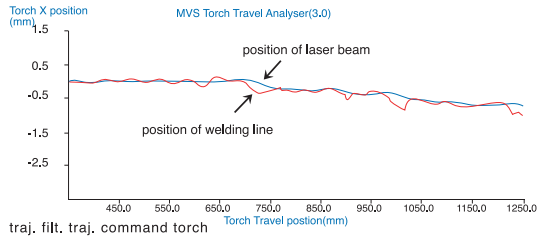
그림 13. Deviation of laser beam and welding line
