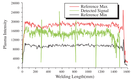
그림 16. Plasma intensity variation at 5 hole defect
