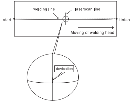
그림 4. Error and deviation in longitudinal welding line of tube
