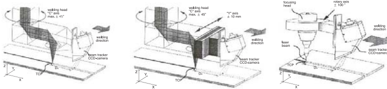
그림 5. Various moving types of laser welding head
