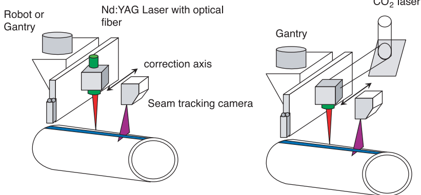
그림 6. Schematic diagram for seam tracking of tube
