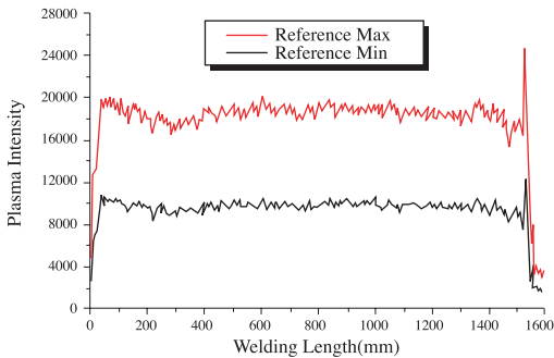
그림 15. Reference Max. and Min. values of plasma intensity
