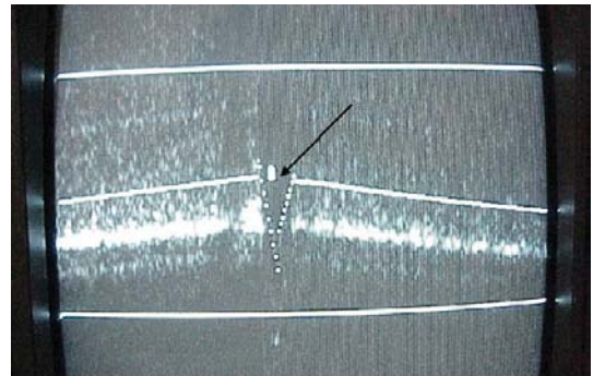
그림 12. Segments profile of tube joint
