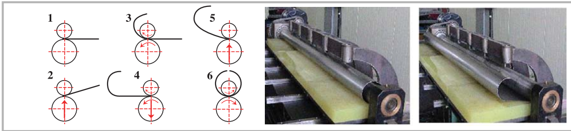
그림 10. 2 roll bending process
