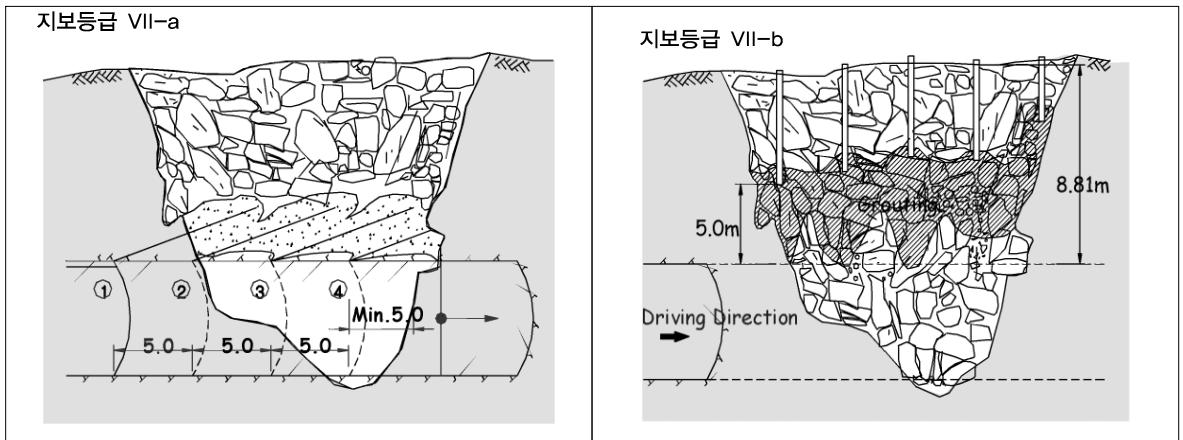
그림 7. 붕괴된 돌리네 통과구간에 대한 지보형식
