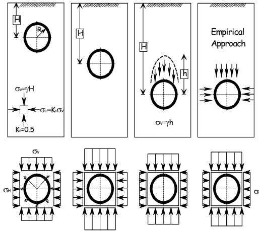
그림 2. Plane Strain Models
