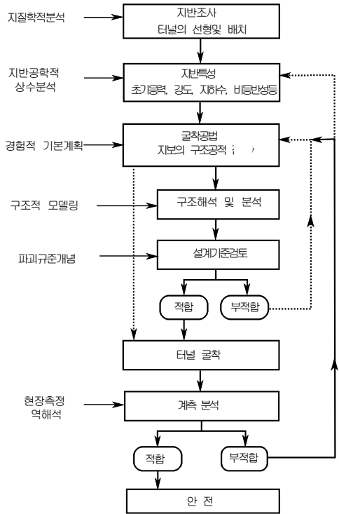
그림 1. 터널의 설계과정 흐름도
