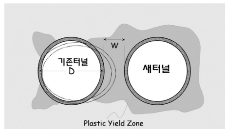
그림 4. 두 평행터널사이의 상호 거동
