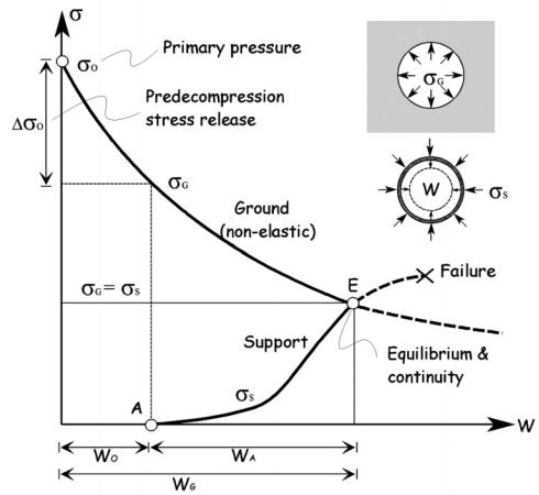
그림 3. Fenner-Pacher Convergence-Confinement 특성
