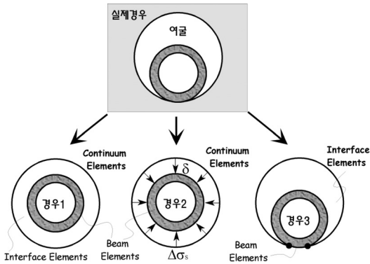
그림 10. 여굴에 대한 모델링
