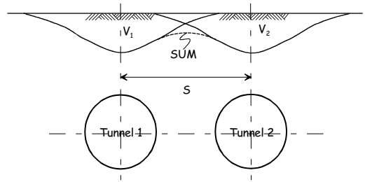
그림 11. 근접터널에 있어서 중첩방법에 의한 지표침하
