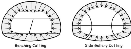
그림 8. 굴착방법에 따른 터널의 변형 비교 (수치해석결과)
