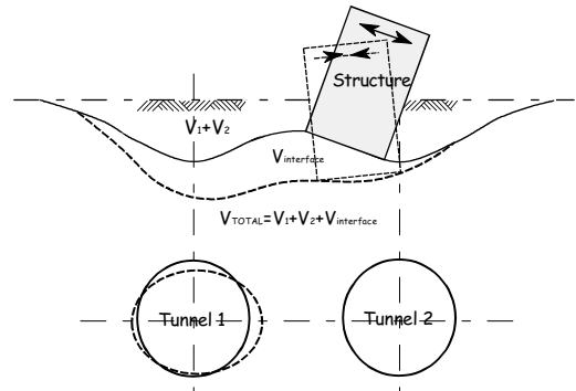
그림 12. 근접터널에 있어서 중첩방법에 의한 지표침하
