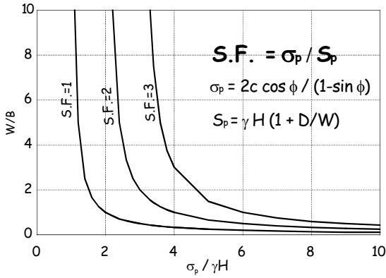
그림 6. 안전율 (S.F.)에 따른 W/B와 강도비 관계곡선
