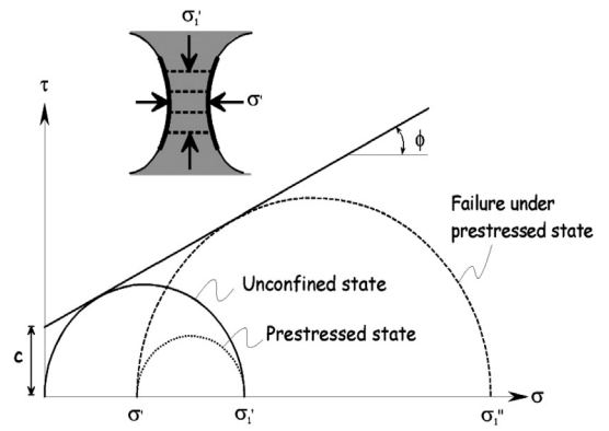
그림 7. 지반의 응력상태 (Prestress 전후)
