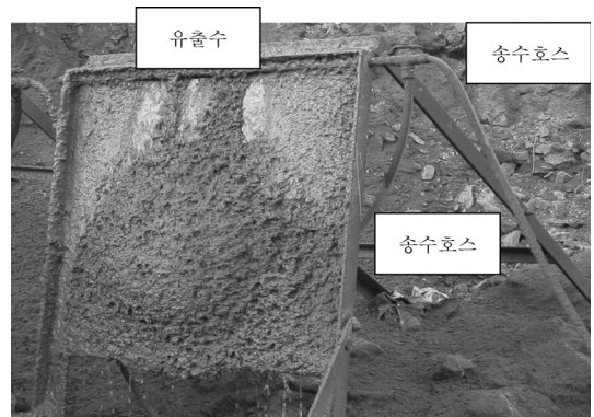
사진 2. 용수부 부착성능시험
