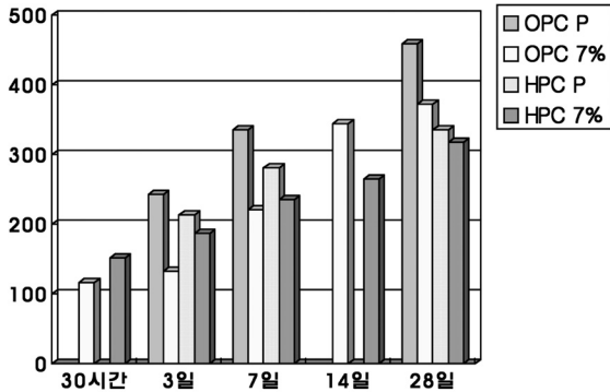
그림 1 압축강도 시험 결과
