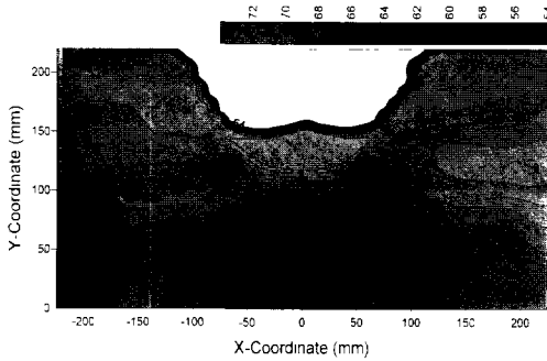
그림 7 모형지반의 최종 함수비 분포 I
