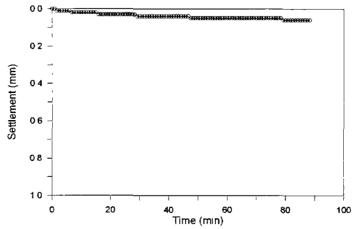
(c) 배면성토부의 시간-압밀침하 관계곡선 그림 11 안정성 검토 모형실험 결과
