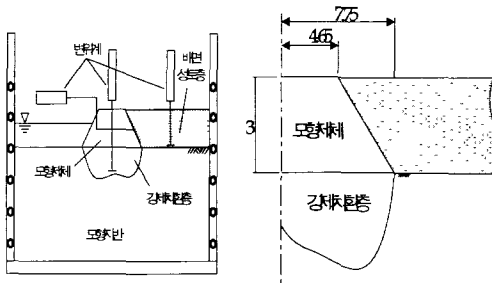
그림 4 안정성 검토 모형실험 개요
