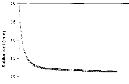
(b) 제체의 연직변위
