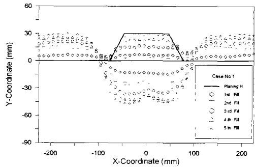
그림 5 모형지반의 성토단계별 침하형상 I
