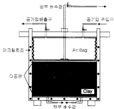
그림 2 강제압밀에 의한 시료성형
