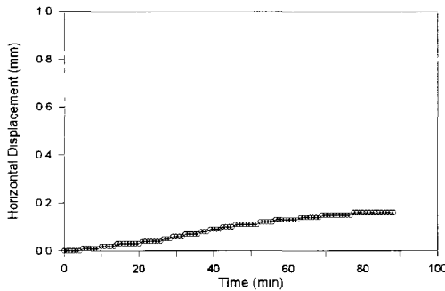
(a) 제체의 수평변위
