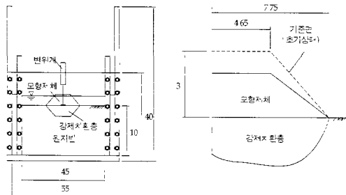
그림 3 강제치환 특성시험 개요
