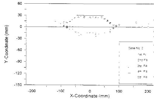
그림 8 모형지반의 성토단계별 침하형상 II
