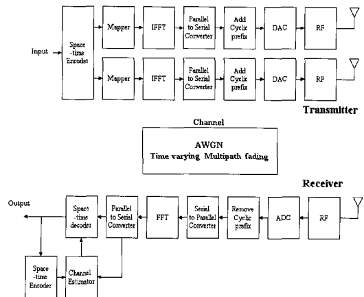
[그림 1] STTC를 이용한 OFDM 시스템
