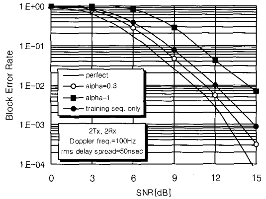
[그림 11] Block Error Rate 성능( f_d = 100\text{Hz} , rms delay spread = 50nsec)
