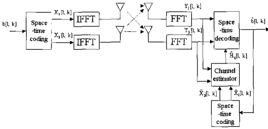
[그림 4] 송신 다이버시티를 가진 OFDM 시스템의 구성도
