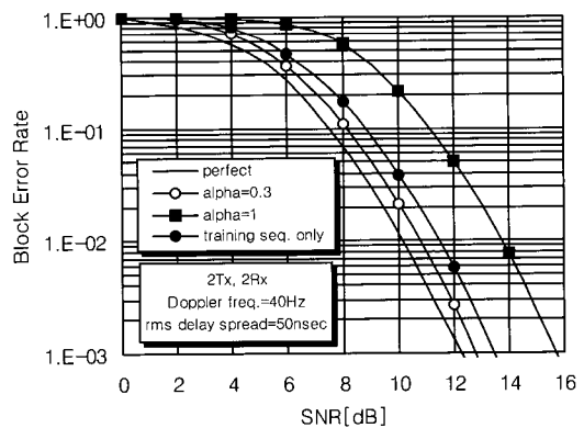
[그림 7] Block Error Rate 성능( f_d = 40\text{Hz} , rms delay spread = 50nsec)
