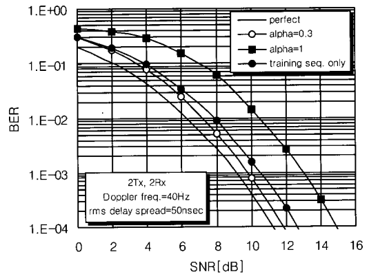
[그림 6] BER 성능( f_d = 40\text{Hz} , rms delay spread = 50nsec)
