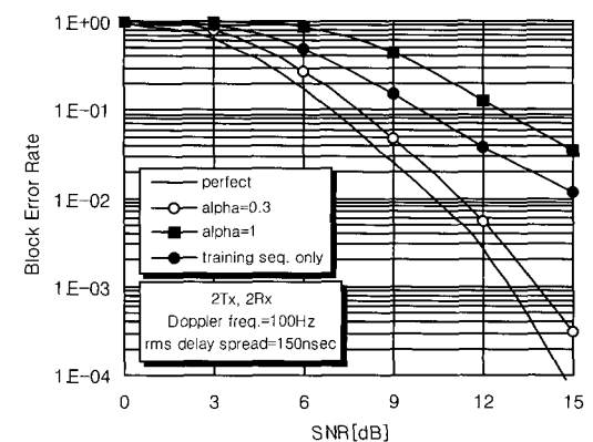
[그림 13] Block Error Rate 성능( f_d = 100\text{Hz} , rms delay spread = 150nsec)
