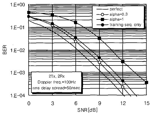
[그림 10] BER 성능( f_d = 100\text{Hz} , rms delay spread = 50nsec)
