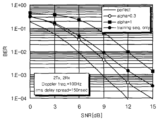
[그림 12] BER 성능( f_d = 100\text{Hz} , rms delay spread = 150nsec)
