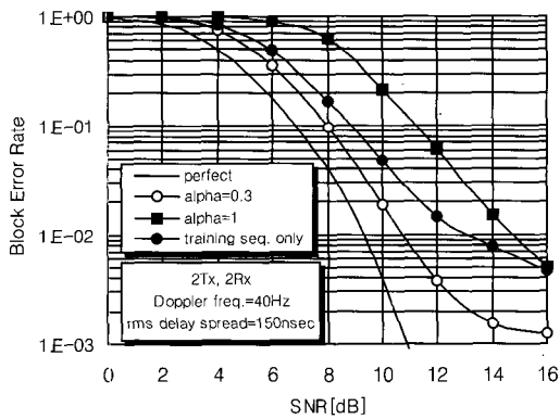
[그림 9] Block Error Rate 성능( f_d = 40\text{Hz} , rms delay spread = 150nsec)
