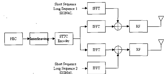
[그림 3] IEEE 802.11a에 STTC를 적용하기 위한 송신기 구조
