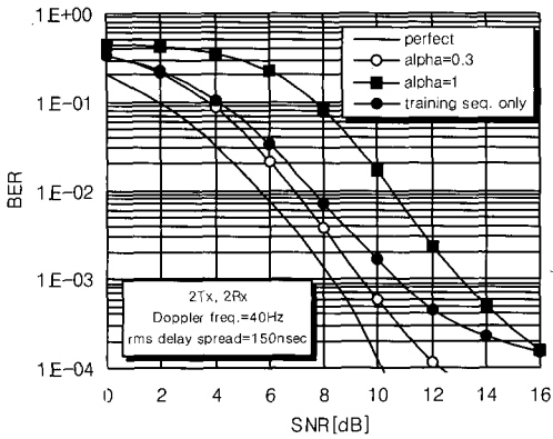
[그림 8] BER 성능( f_d = 40\text{Hz} , rms delay spread = 150nsec)
