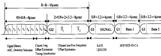
[그림 2] IEEE 802.11a의 프레임 구조
