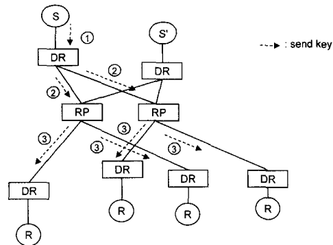
(그림 7) 데이터 전송 과정
