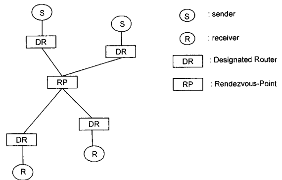
(그림 1) PIM-SM 그룹키 관리 구조
