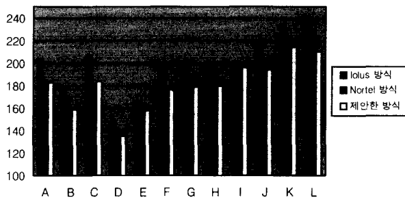
(그림 9) 데이터 전송 최대소요시간
