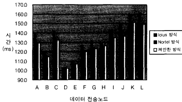
(그림 8) 데이터 전송 평균시간
