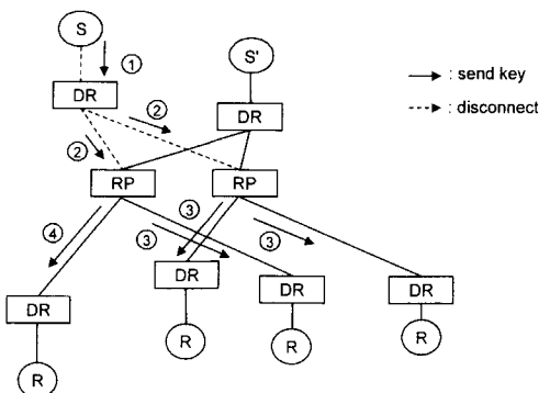
(그림 3) 송신자의 그룹 탈퇴 과정
