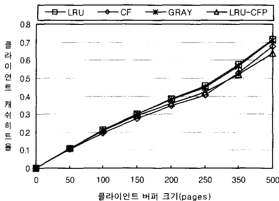
(그림 6) 클라이언트 캐쉬히트율
