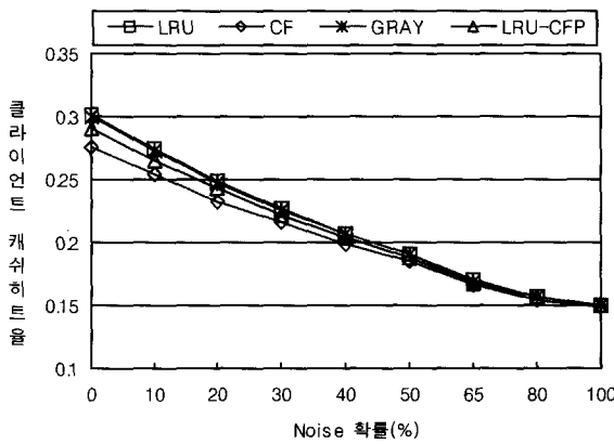
(그림 9) 클라이언트 캐시히트율
