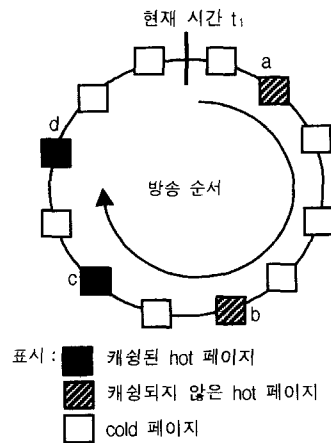
(그림 2) LRU-CFP 기법의 캐쉬 관리
