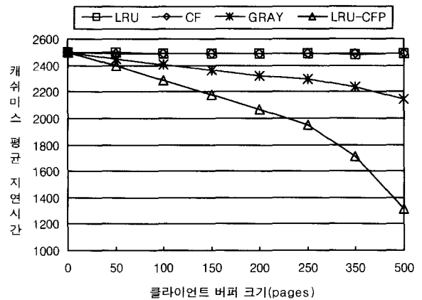
(그림 7) 캐쉬미스시의 평균 지연시간(ticks)
