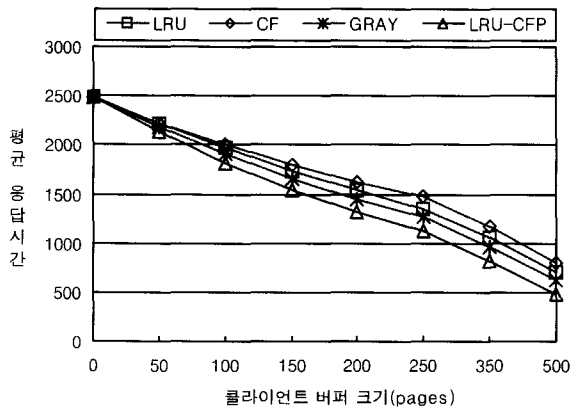
(그림 4) 평균 응답시간(ticks)
