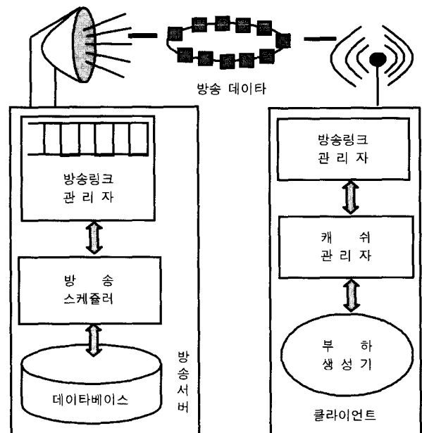
(그림 3) 성능 평가 모델
