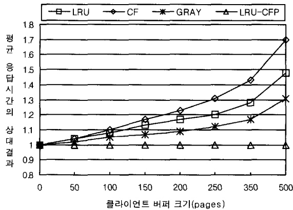
(그림 5) 평균 응답시간의 상대결과
