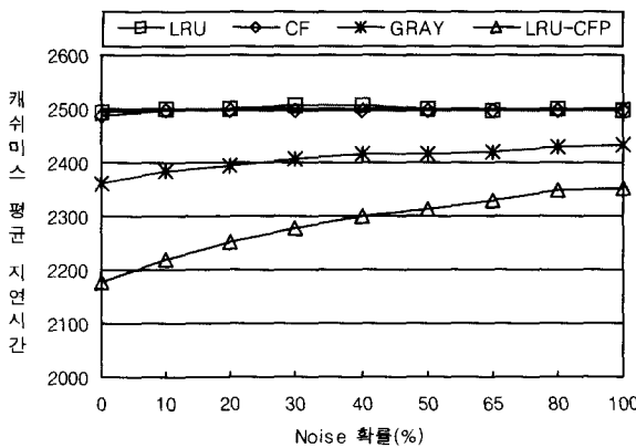
(그림 10) 캐시미스의 평균지연시간
