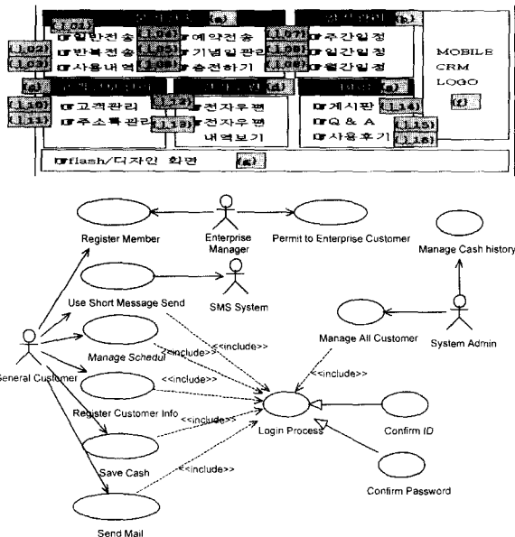
(그림 6) 스토리보드와 Use Case Diagram
