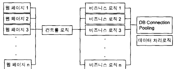
(그림 2) 어플리케이션 중심의 설계방법
