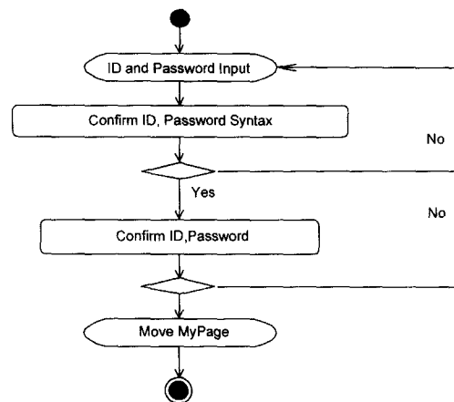
(그림 7) 회원인증 Use Case에 대한 Activity Diagram
