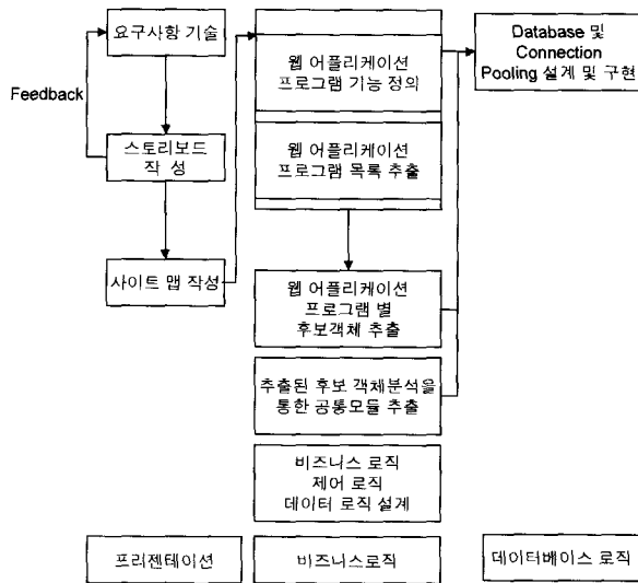
(그림 1) 개발 프로세스
