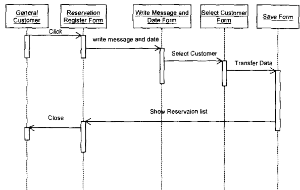
(그림 8) 문자예약 전송 시퀀스 다이어그램
