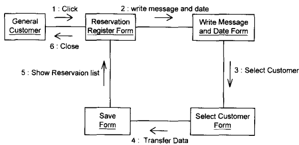
(그림 9) 문자예약 전송 콜러보레이션 다이어그램
