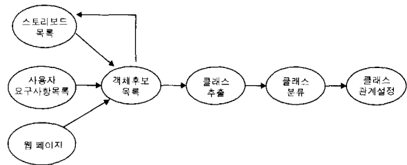
(그림 10) 클래스 추출 프로세스
