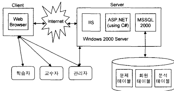
(그림 3) 전체 시스템 구성
