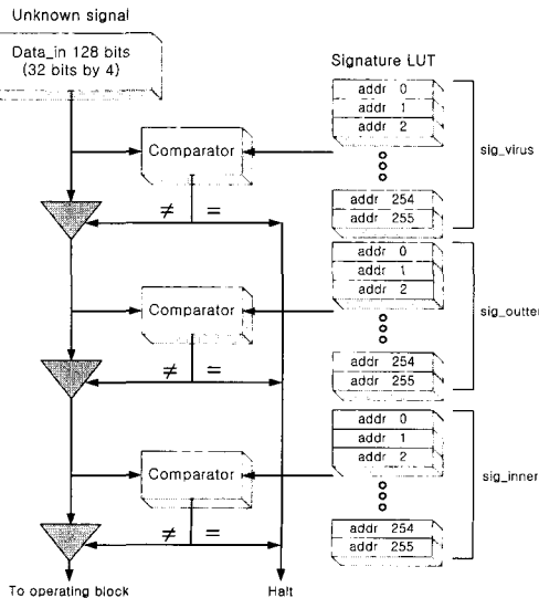
그림 3. 제안된 통합 IDS 게이트웨이 기능 블록도
