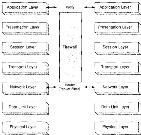
그림 1. OSI 계층과 방화벽
