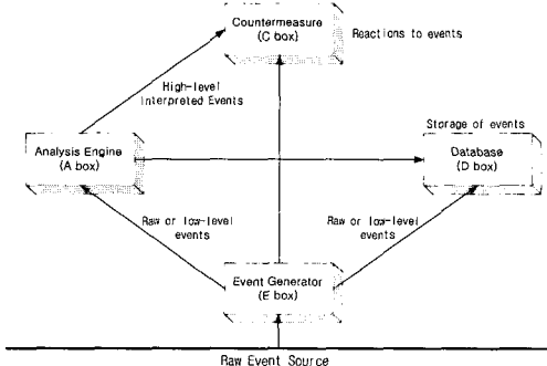
그림 2. CIDF의 IDS 개념도
