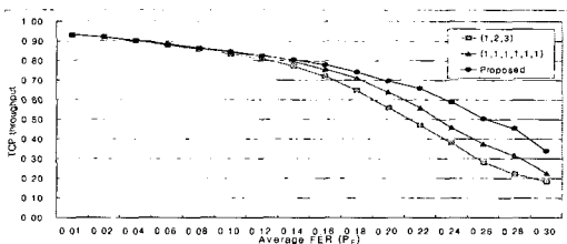
그림 10. f_d T = 0.01 인 페이딩 채널에서 FER에 따른 TCP 수율 Fig. 10 TCP throughput vs. FER over fading channel with f_d T = 0.01
