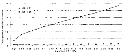
그림 9. 프레임 에러 버스트 평균 길이 Fig. 9 Average length of frame error bursts
