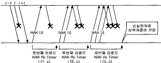
그림 3. (1,2,3) 에러복구 방법(IS-707 RLP) Fig. 3 N(1,2,3) error recovery scheme(IS-707 RLP)
