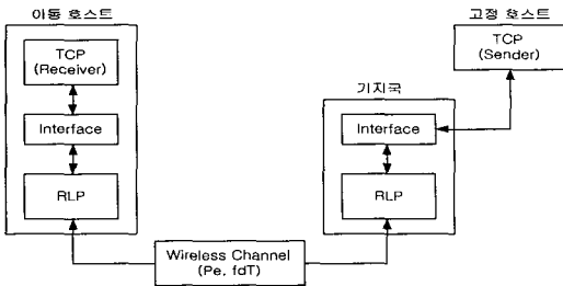
그림 8. TCP/RLP 시뮬레이션 모델 Fig. 8 TCP/RLP simulation model
