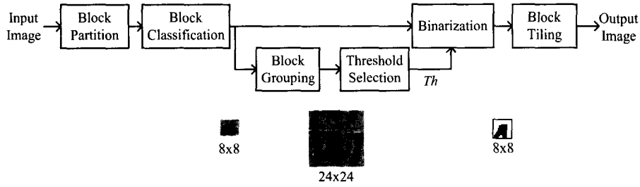
그림 3. 블록적응 이진화 과정 Fig. 3. Procedure of BAB.
