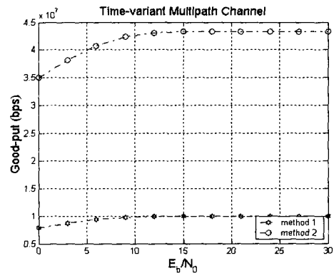
그림 7. 시변 채널에서 방법 1과 방법 2의 Good-put 성능.
