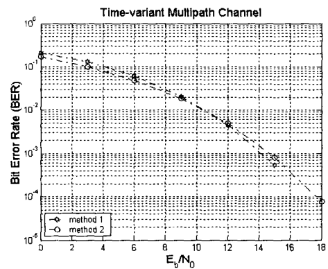
그림 6. 시변 채널에서 방법 1과 방법 2의 비트오율 성능.
