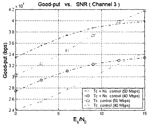
그림 4. 채널 3에서 N_s 와 T_c 조절과 T_c 조절의 비교.
