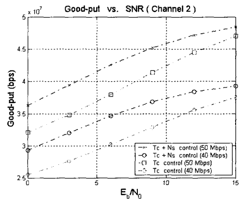
그림 3. 채널 2에서 N_s 와 T_c 조절과 T_c 조절의 비교.
