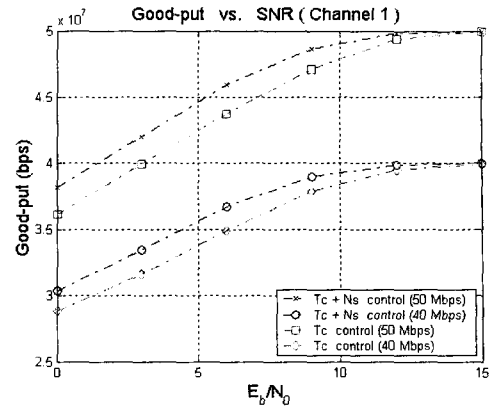
그림 2. 채널 1에서 N_s 와 T_c 조절과 T_c 조절의 비교.
