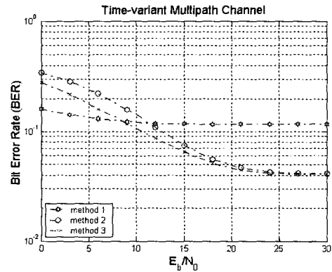
그림 5. 시변 채널에서 세 가지 방법의 비트오율.
