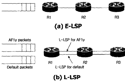
그림 9. E-LSP와 L-LSP의 동작
