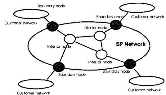
그림 2. DiffServ의 개괄적인 구조
