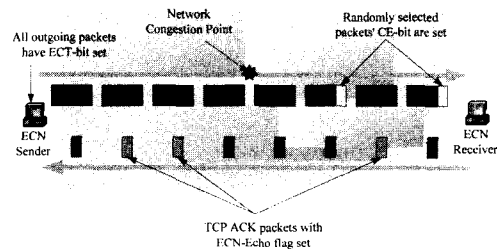
그림 5. 중단간 ECN 동작도
