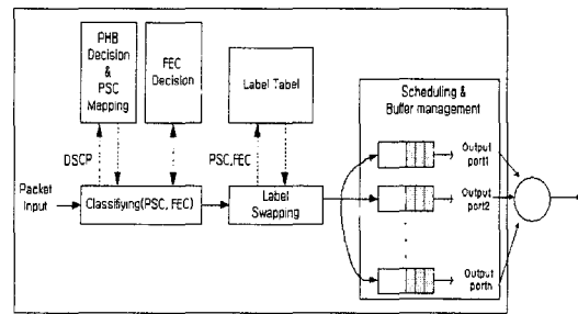
그림 8. DiffServ를 지원하는 MPLS의 동작
