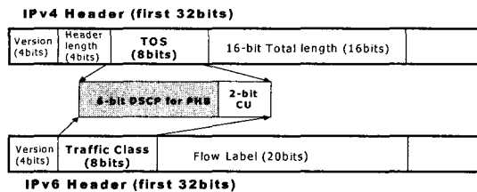
그림 1. DSCP 필드
