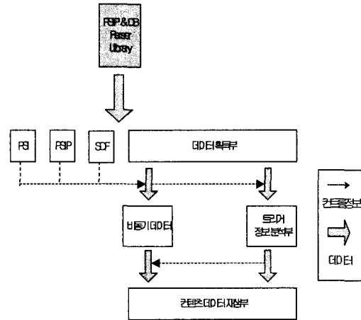
그림 3. 트리거 정보를 이용한 비동기 데이터 처리를 위한 시스템 구조
