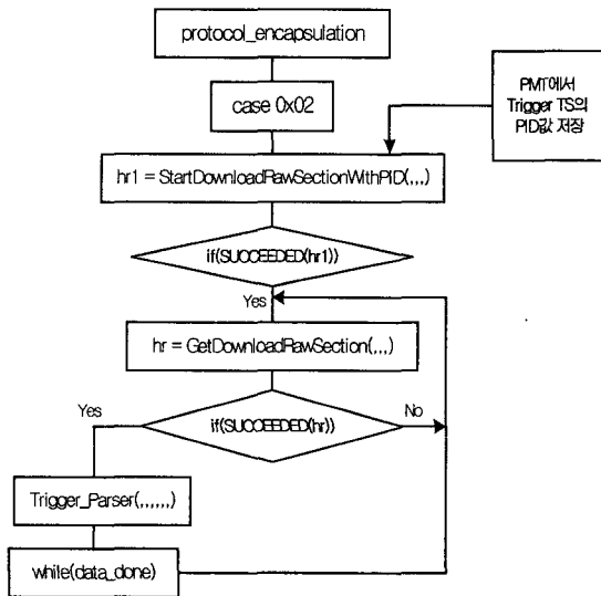
그림 4. 트리거 정보를 이용한 비동기데이터의 동기화 흐름도 Fig 4. Block diagram of asynchronous data synchronization by using trigger information
