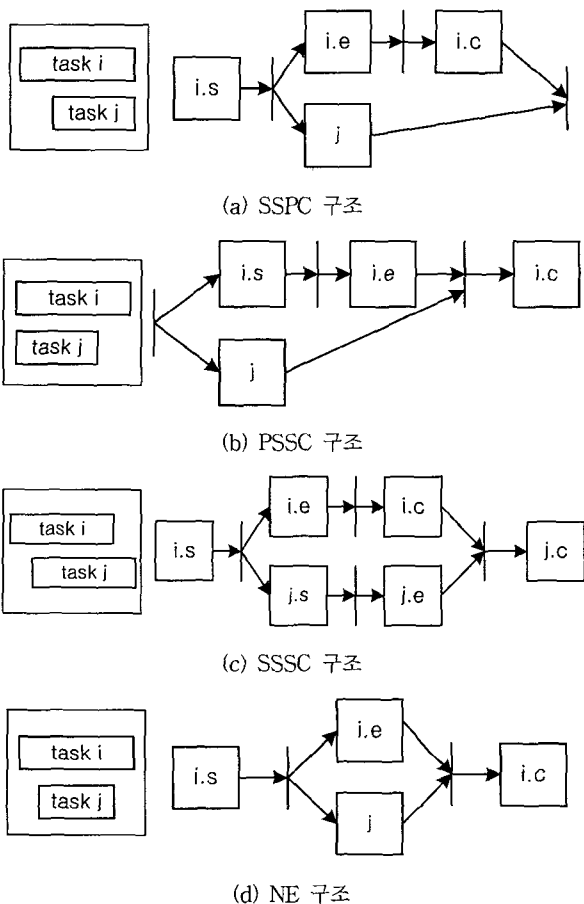
(그림 3) 병행처리 구조의 EMFG 표현
