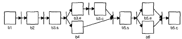
(그림 4) 다양한 병행처리의 예
