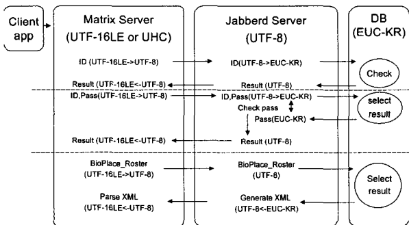
(그림 22) 한글 데이터의 처리 과정
