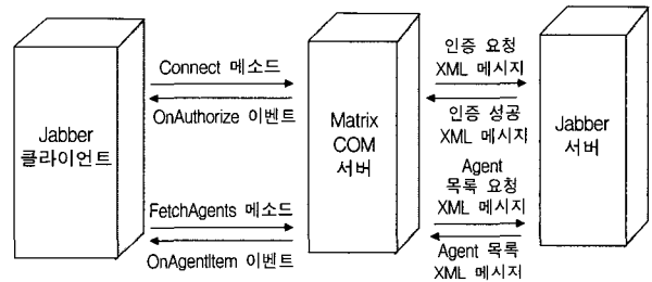
(그림 16) Matrix COM의 구동 원리
