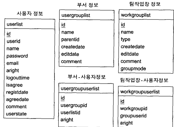
(그림 5) 메신저 시스템과 관련된 BioPlace의 데이터베이스 테이블
