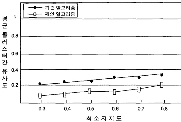
(b) 클러스터간의 유사도
