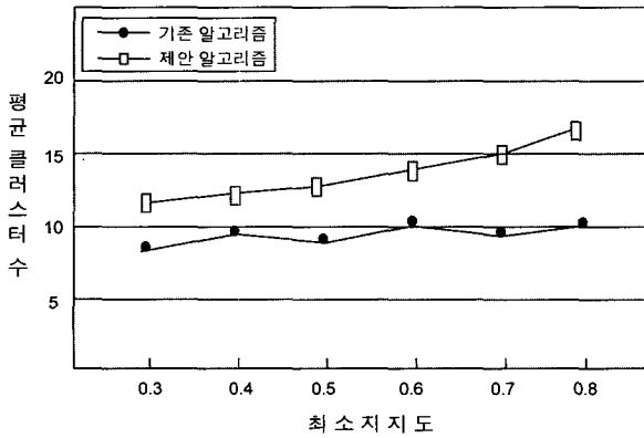
(그림 3) 평균 클러스터 수
