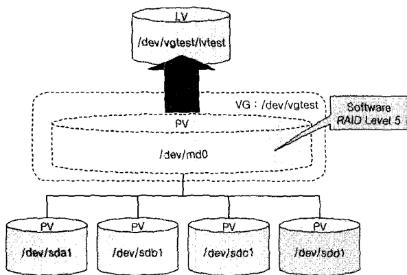
(그림 5) 소프트웨어 RAID 레벨 5와 LVM이 적용된 저장 장치
