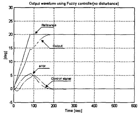
(a) 외란이 없는 경우 (a) No disturbance
