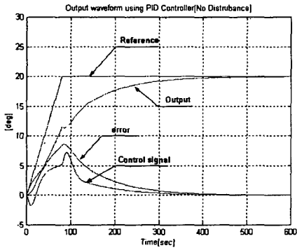
(a) 외란이 없는 경우 (a) No disturbance
