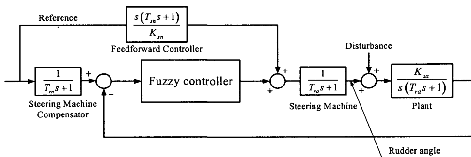
그림 2. 퍼지 제어를 사용한 선박시스템 Fig. 2. System of Ship using Fuzzy Controller
