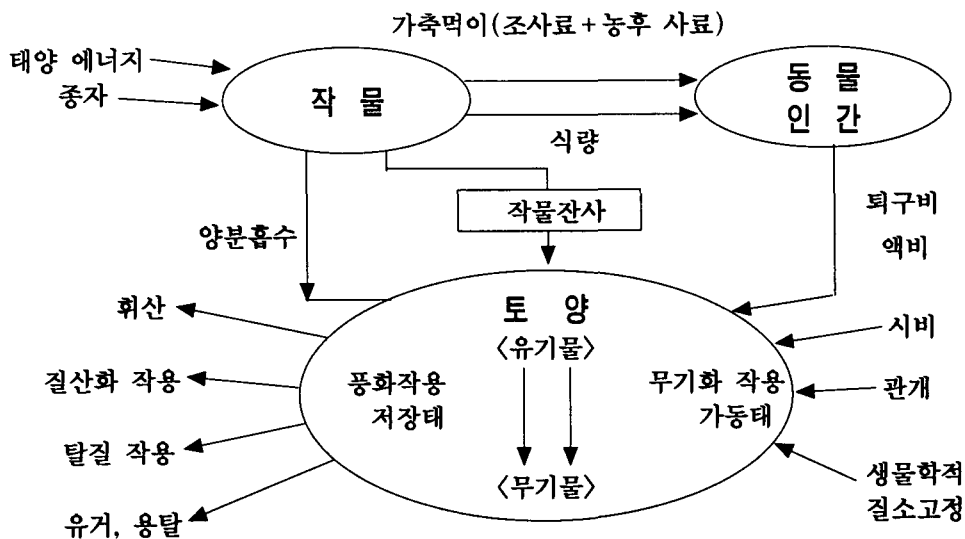
〈그림 1〉 농업생태계에서의 물질순환
