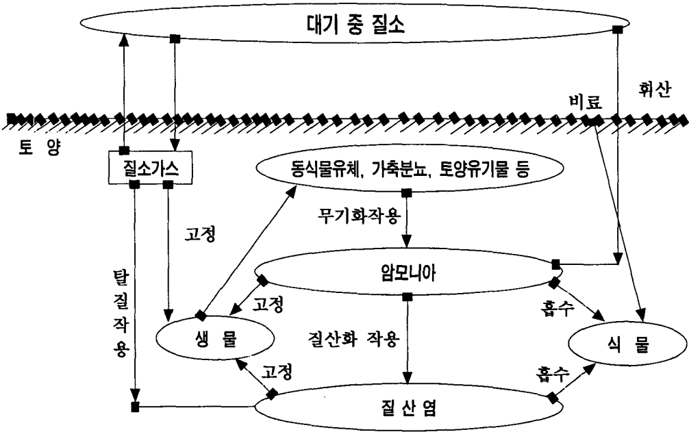
<그림 2> 토양에서의 질소 흐름(Tivy, 1990)
