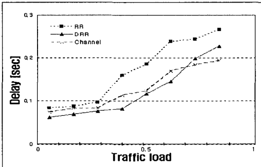
b) 지연시간
