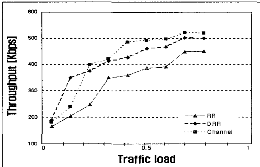
a) 처리율
