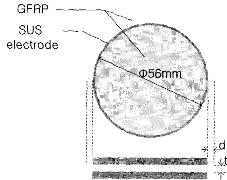
그림 2. 솔레노이드형 턴간 전극 배치.
