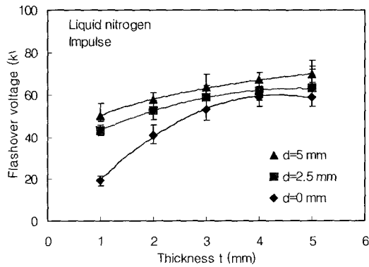
그림 6. Impulse 연면방전 전압에 미치는 두께의 영향. Fig. 6. Effect of thickness on impulse flashover voltage.
