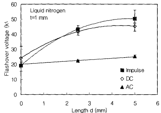
그림 7. 연면방전 전압에 미치는 길이의 영향. Fig. 7. Effect of surface length on flashover voltage.
