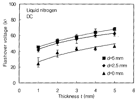
그림 5. DC 연면방전 전압에 미치는 두께의 영향. Fig. 5. Effect of thickness on DC flashover voltage.
