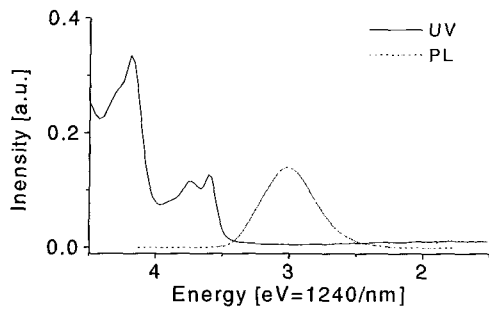
그림 5. PVK의 UV/visible과 PL 분광분석. Fig. 5. UV/visible and PL spectra of PVK.
