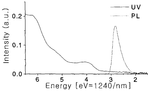
그림 2. PBD의 UV/visible과 PL 분광분석. Fig. 2. UV/visible and PL spectra of PBD.
