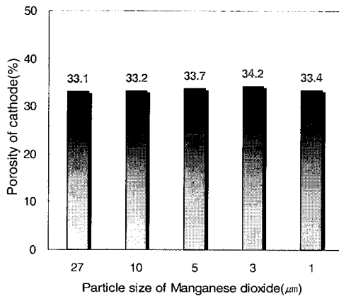
그림 9. 촉매입자 크기에 따른cathode의 기공율. Fig. 9. Porosity as a function of particle size of catalyst in cathode.
