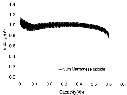
그림 6. GSM 펄스방전에 의한 전압 패턴.
