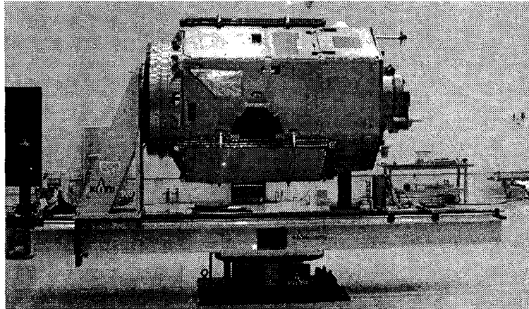
그림 3. 다목적 실용위성 2호 질량특성 측정 - 수평측.
