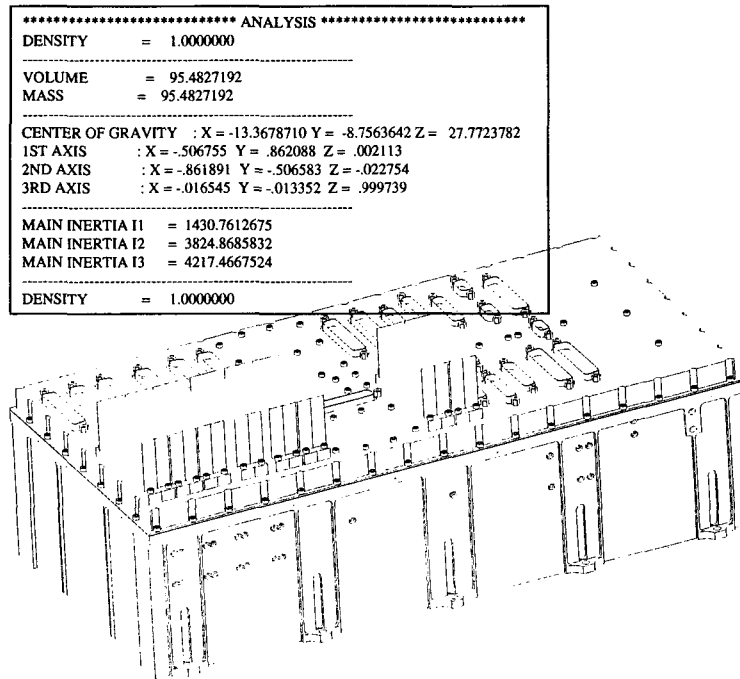
그림 1. CATIA에서의 단품 관성 모멘트 해석 결과.
