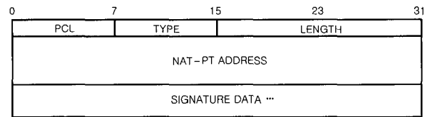
(그림 4-6) NAT-PT 서명 페이로드 포맷
