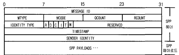
(그림 4-3) 확장된 SPP 메시지 헤더 포맷
