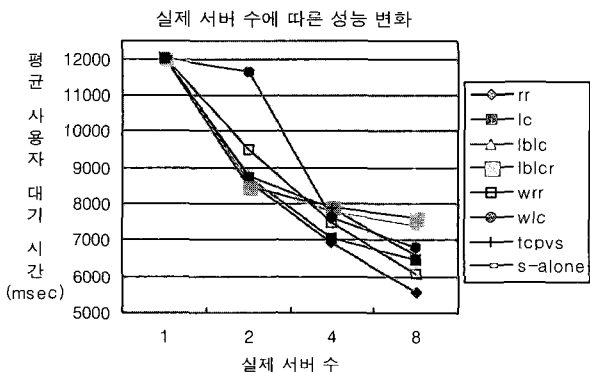
(그림 9) 실제 서버 수에 따른 성능 변화
