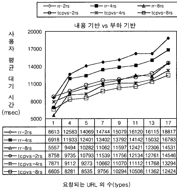
(그림 10) 요청 type 수에 따른 성능 변화
