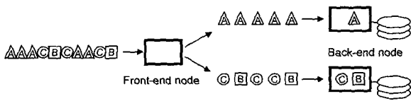
(그림 2) 내용 기반 요청 분배 알고리즘
