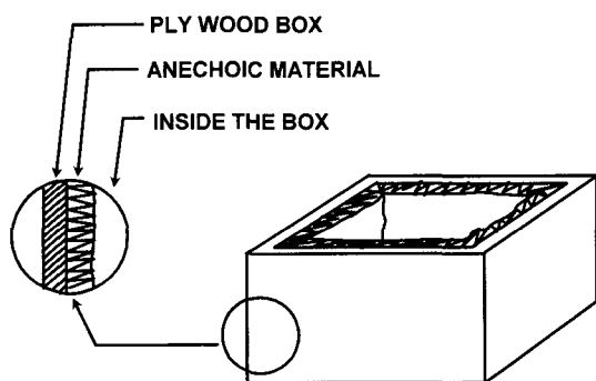
Fig. 3 Anechoic box
