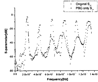
그림 8. PBG의 주파수 응답 특성 Fig 8. Frequency response of PBG
