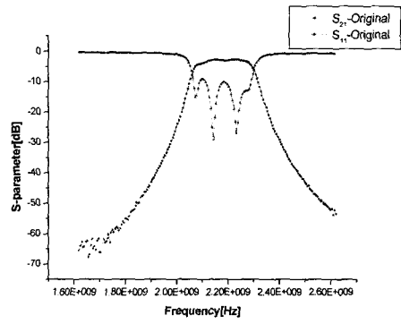
그림 2. 필터의 주파수 응답 곡선(협대역) Fig 2. Filter response (narrow view)
