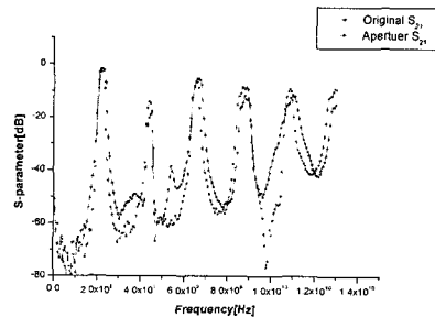
그림 6. Aperture의 주파수 응답특성(광대역, 21m) Fig 6. Frequency response of Aperture (wide view, 21m)
