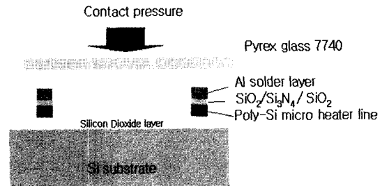
Fig. 7. FP scheme 미세 가열기를 이용한 접합 과정 단면도.
