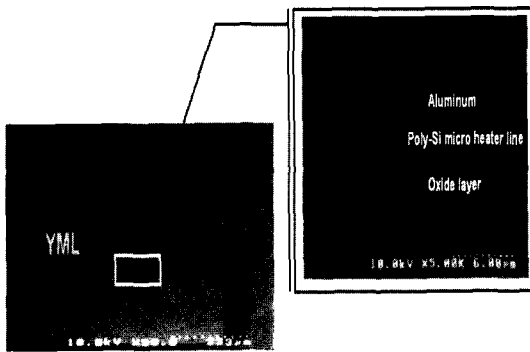
Fig. 5. FP scheme 미세 가열기의 공정 후 SEM 형상.
