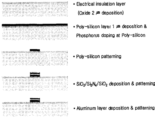
Fig. 4. FP scheme 미세 가열기의 제작 공정 순서.
