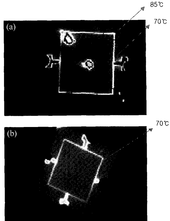
Fig. 6. (a) conventional scheme의 미세 가열기에 IR camera 실험 결과. (b) FP scheme 미세 가열기의 IR camera 실험 결과.
