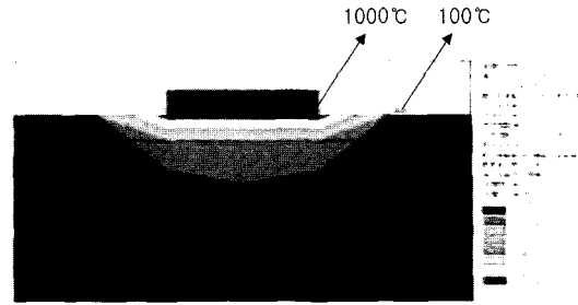
Fig. 1. 미세가열기의 2차원 열전도 시뮬레이션 결과.
