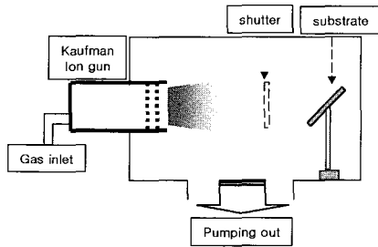
그림 1. IB 조사 시스템.
