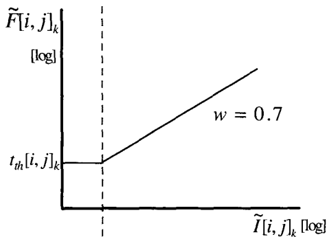
그림 3. 주파수 마스킹 함수 Fig. 3. Frequency masking function
