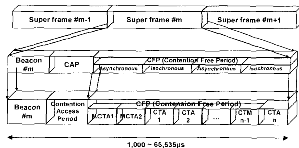
그림 8. IEEE802.15.3 Super Frame의 구조
