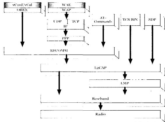
그림 7. 블루투스의 프로토콜 stack
