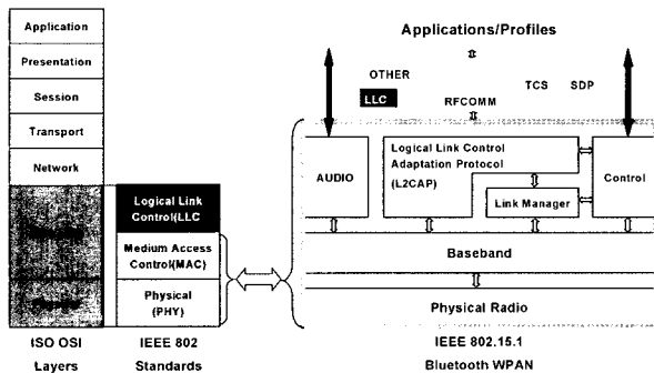
그림 6. OSI 7 Layer & 블루투스
