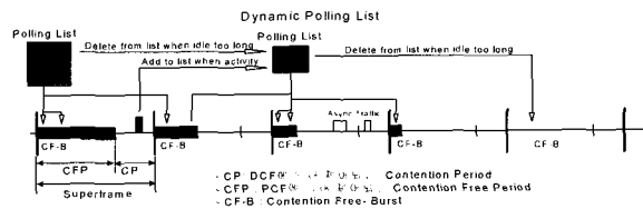
그림 4. IEEE802.11 PCF 방식
