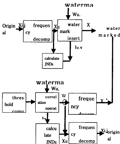
그림 3.1 이미지 적응 워터마크의 일반적인 블록 다이어그램
