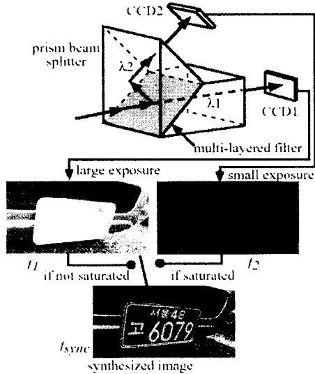
그림 2. 제안된 인식 시스템의 원리 Fig 2. The principles of the proposed sensing system
