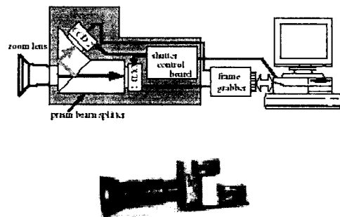
그림 3. 제안된 인식 시스템의 구조 Fig 3. The structure of the developed sensing system
